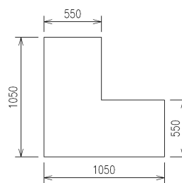
RH3/P(L) Rohová skřínka pravoúhlá - vnější roh
