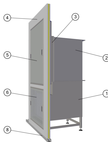
1 - Stěnový nástavec; 2 - Nástavec TROX; 3 - Límec; 4 - Panel tl. 60mm; 5 - Revizní poklop, 6 - Mřížka, 8 - Basic profil
