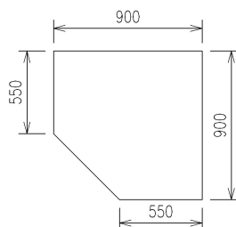
RH2 Rohová skrinka so skoseným rohom
