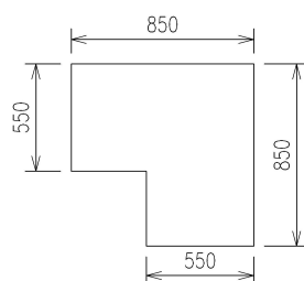
RH1 Rohová skrinka pravoúhlá - vnútorný roh
